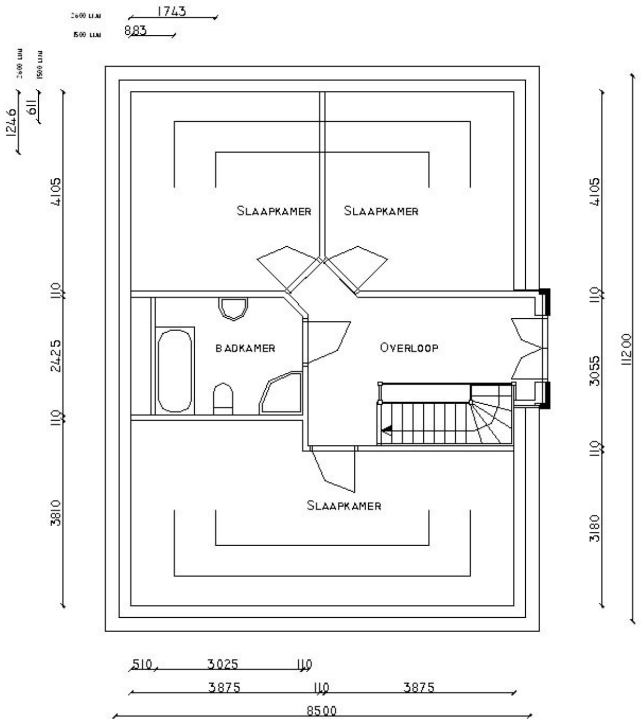
VERD. WONING 8.5 x 11.20 M TYPE HEEMSTEDÉ
